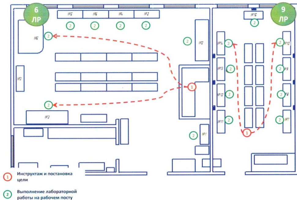
Целевая диаграмма спагетти перемещений при выполнении выполнения лабораторных работ по разделу электрооборудование автомобилей
