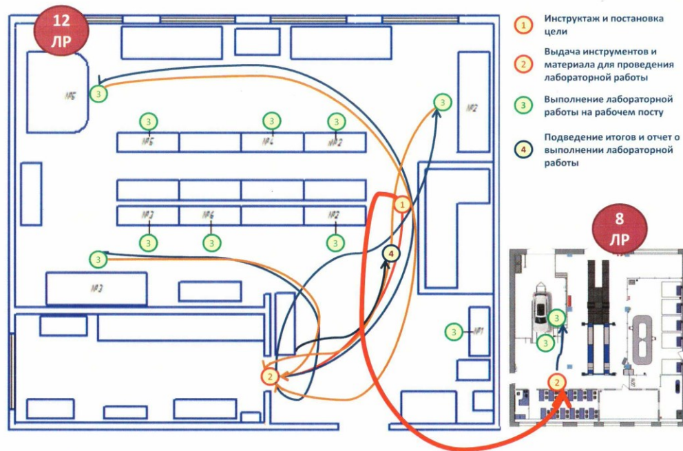
Диаграмма спагетти текущих перемещений при выполнении выполнения лабораторных работ по разделу электрооборудование автомобилей
